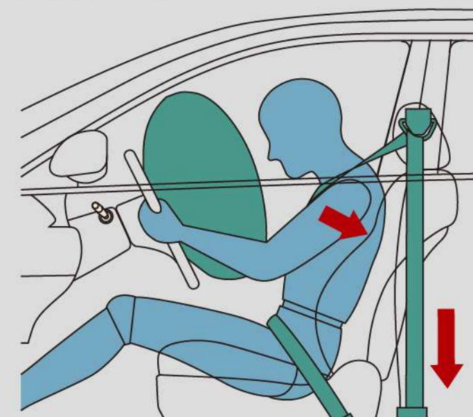
預縮作用
