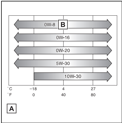
A 下次更換機油前預期的氣溫範圍
