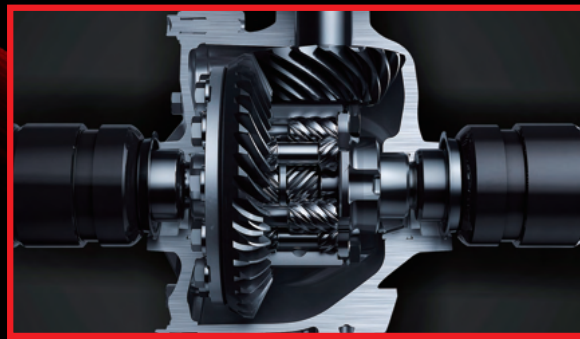
Torsen® LSD 前、後軸限滑差速器
