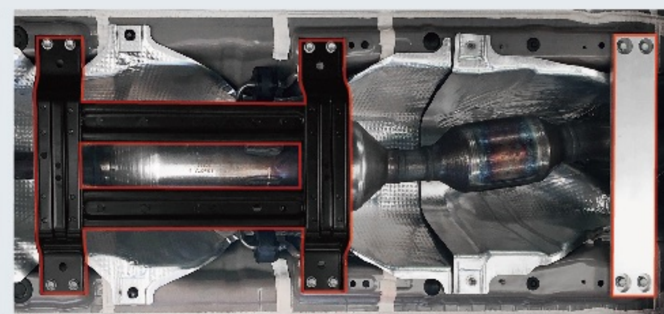
GR SPORT 底盤強化支架
