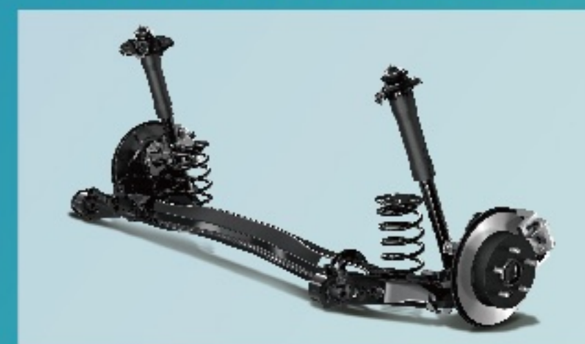
全新 TNGA 扭力桿式後懸吊
