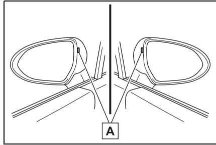
A BSD/RCTA 接近指示燈
