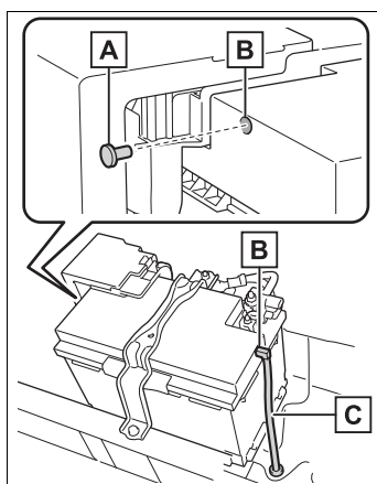
A 排氣孔塞
