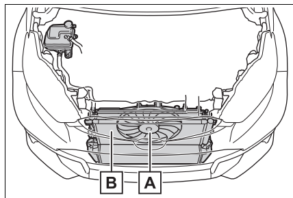
A 冷卻風扇
