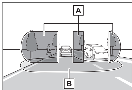
A 遠光燈照亮範圍
